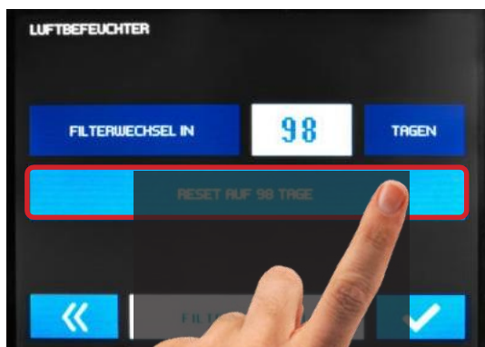
Abb. 6.3.2.7: Filterwechselanzeige zurücksetzen
