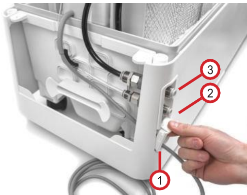
Abb. 7.4.1.2: Seitendeckel öffnen
