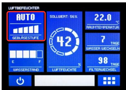
Abb. 5.1.1: Anzeige Gebläsestufe
