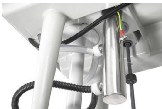
Abb. 8.1.2.8: UV-Entkeimungseinheit, komplett
